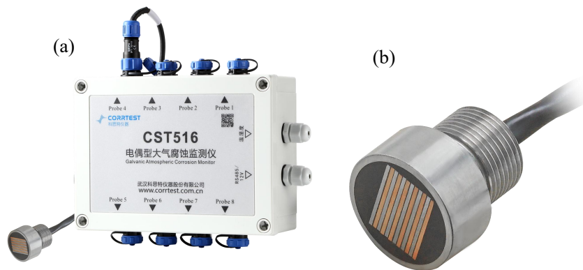
图 1 (a) 电偶型大气腐蚀监测仪；(b) ACM 传感器
