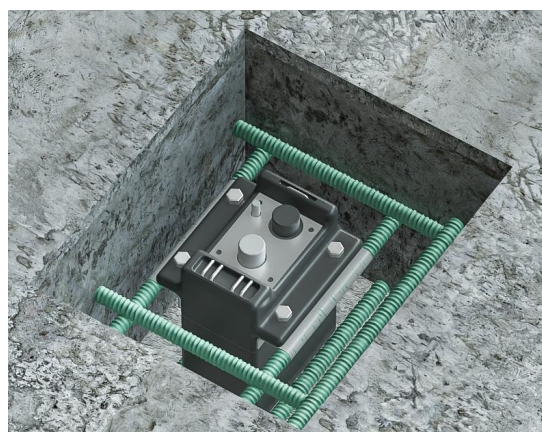
图 2. CST710 一体式混凝土腐蚀监测仪安装示意图
