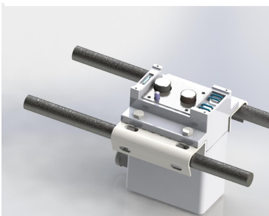
图 2. CST710 一体式混凝土腐蚀监测仪安装示意图
